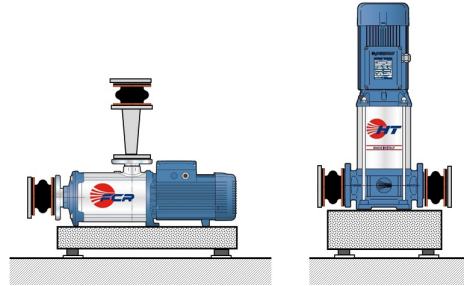
Рис. 6.5 – Приклад встановлення для зменшення вібрації та шуму
