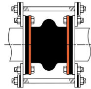
Рис. 6.6 – Приклад гумового з'єднання з анкерними шпильками
