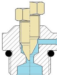
Рис. 7.2 – Пробка стравлювання повітря V
