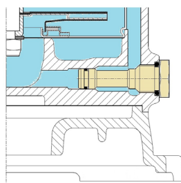
Рис. 7.3 – Зливна пробка D
